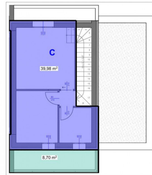
PIANO PRIMO - VILLA "C"
