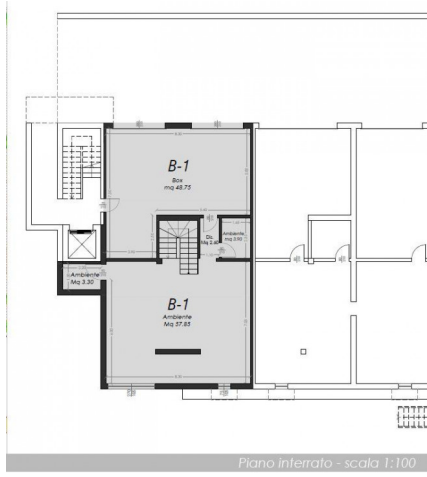
Piano interrato - scala 1:100
