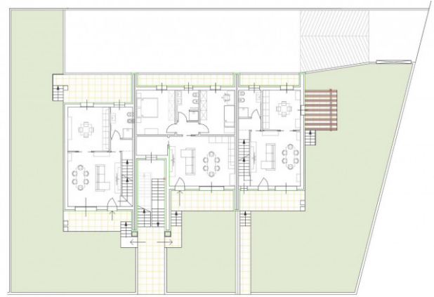
PIANO RIALZATO
