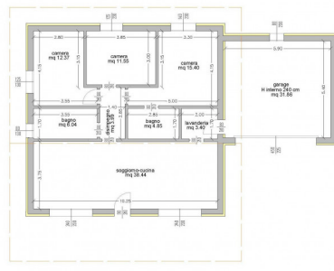
Pianta piano terra - scala 1:100
